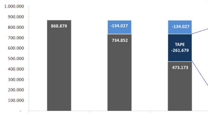
Emissioni di CO 2 per il Settore Trasporti negli anni 1991, 2005, 2020. (ton/anno)
